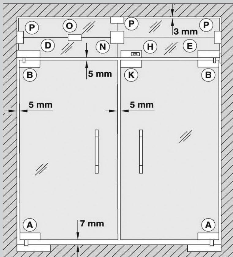
Двустворчатые двери
