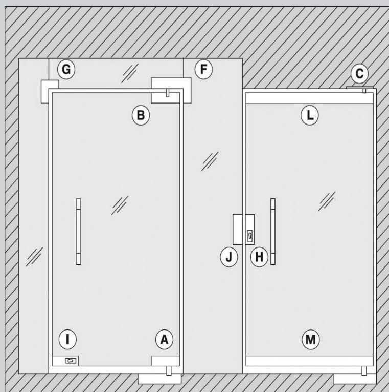
Одностворчатые двери
